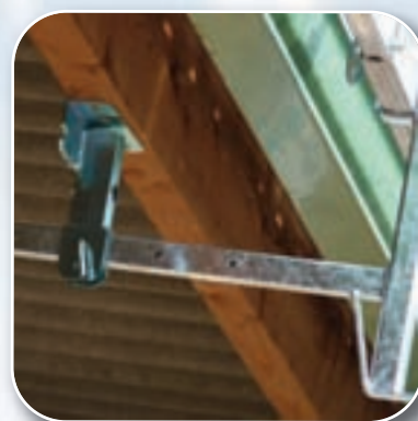
PANNE BOIS avec 4 vis torx Dimos ø8x100
